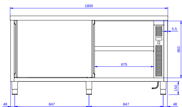
Zepředu
